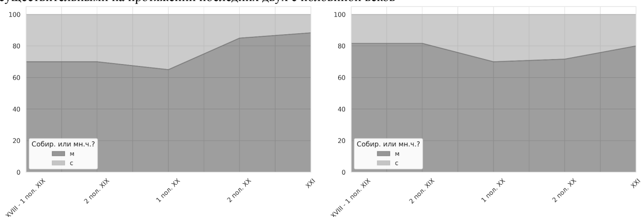
Рис. 5. Доля (%) употреблений среди (слева) и в кругу (справа) с собирательными существительными на протяжении последних двух с половиной веков
