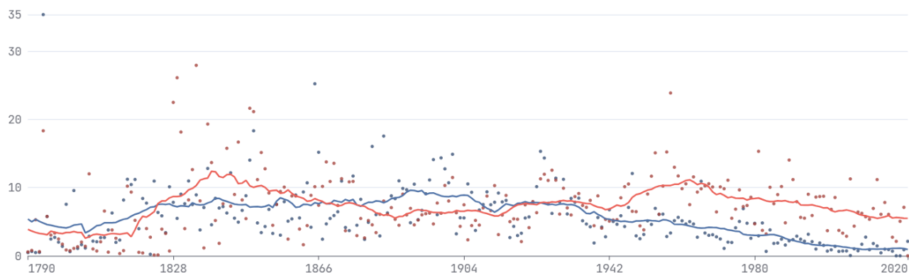
Рис. 6. Частотность посреди (красным) и среди (синим), управляющих (в терминологии корпуса — управляемых) словоформами комнаты|улицы|леса|моря|поля|двора за последние 230 лет. График построен на ruscorpora.ru , сглаживание — 10.
