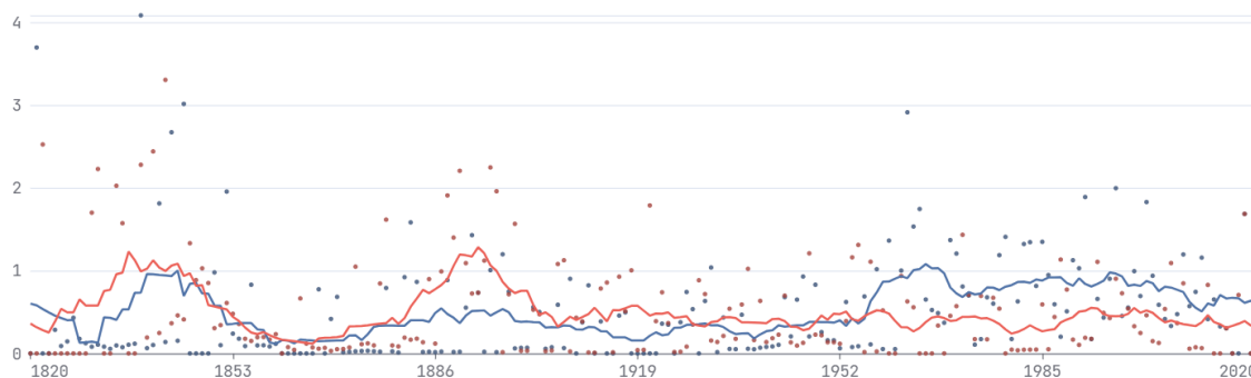
Рис. 1. Частотность сочетаний в семейном кругу (красным) и в кругу семьи | в кругу семейства (синим) за последние 200 лет, график построен на ruscorpora.ru . Сглаживание — 6.
