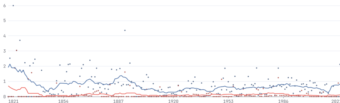
Рис. 2. Частотность сочетаний в дружеском|товарищеском кругу (красным цветом) и в кругу друзей|товарищей (синим цветом) за последние 200 лет, график построен на ruscorpora.ru . Сглаживание — 6.
