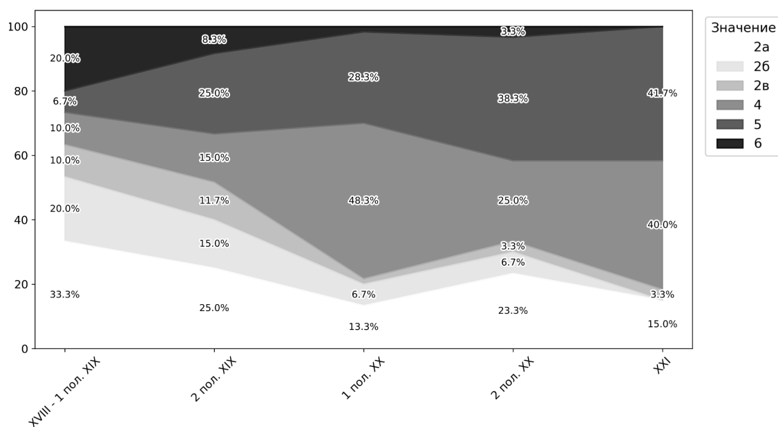
Рис. 4. Доля различных значений среди (%) на протяжении последних двух с половиной веков
