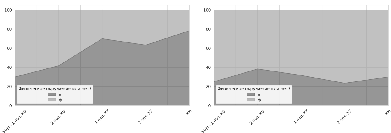
Рис. 3. Доля (%) локативных употреблений среди (слева) и в кругу (справа) на протяжении последних двух с половиной веков
